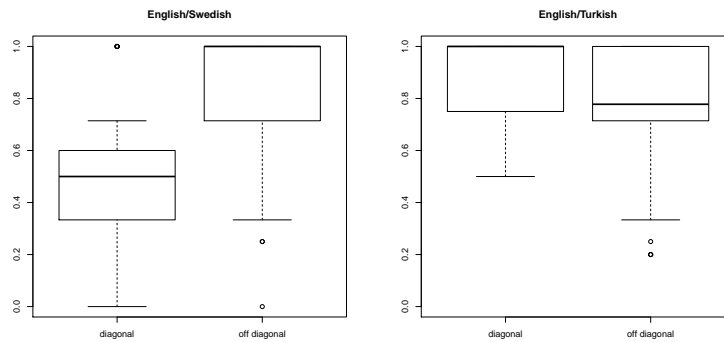
Abbildung 4: Verteilung von Levenshtein-Distanzen
