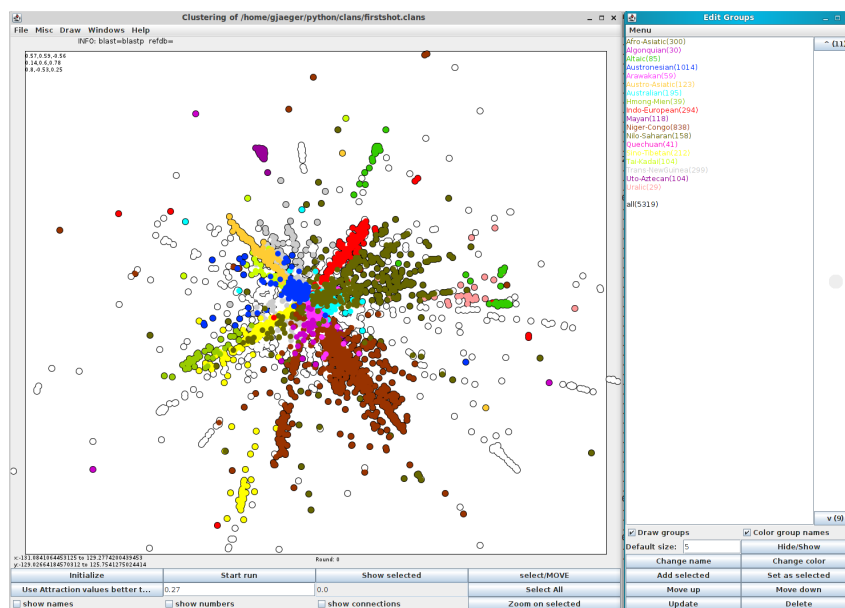
Abbildung 3: Visualisierung der Ähnlichkeiten in ASJP: einfache Levenshtein-Alinierung
